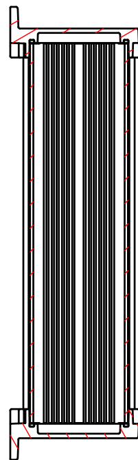
B-B (1:3.5)
