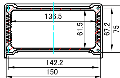
A-A (1:3.5)
