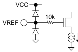
Fig.49 VREF
