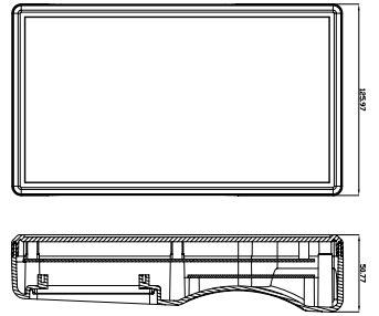
TOP-(NO-LCD)
