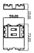
2X2A-BOX
