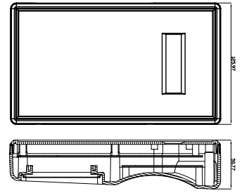
TOP-(NO-LCD)
