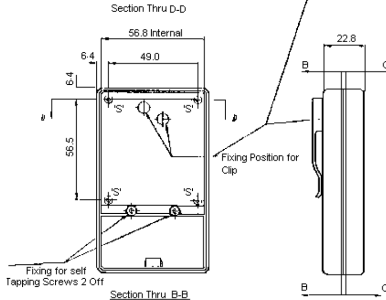
Optional Pocket Clip
